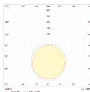
LVK CP55/5
