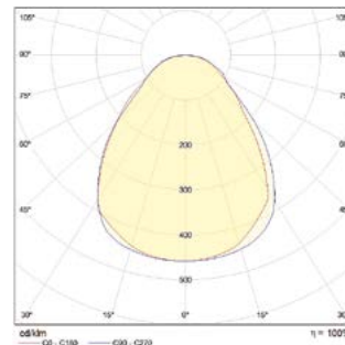
LVK LEDPG40W/4/19
