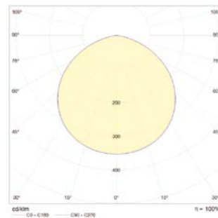
HBO150 LVK
