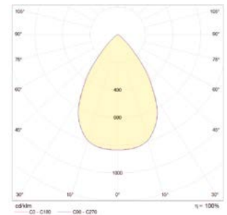
HBO150LG LVK
