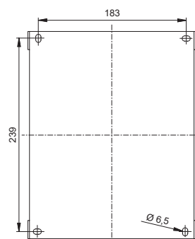
Bohrabmessungen Montageplatte
