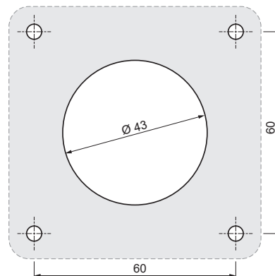
Flansch: 75x75 mm
