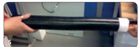
5 Die äußere Schutzhülle positionieren und installieren
