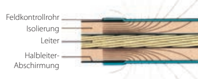
MIT FELDKONTROLLROHR
