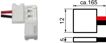
15724000 Einspeisung für 15201...
