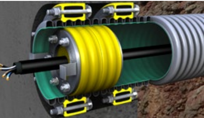
Wandeführung mit Kabu-Seal, Kabu-IN DD und Kabuflex R plus 750 co2ntrol
