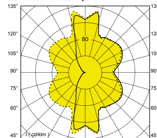
Lichtstärkeverteilung
