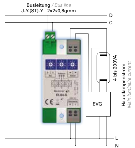
Schaltbeispiel 2: EVG Circuit example 2: EVG
