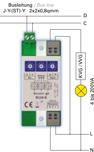
Schaltbeispiel 1: KVG und VVG Circuit example 1: KVG and VVG
