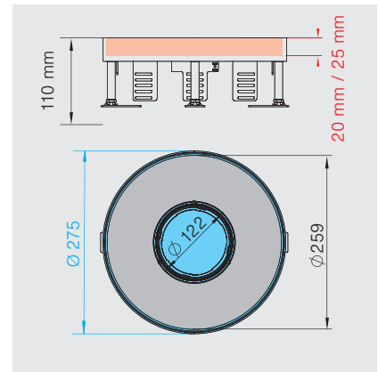
Nenngröße R7, Typ RKFR2 und RKFRN2
