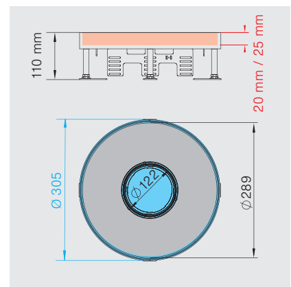
Nenngröße R9, Typ RKFR2 und RKFRN2
