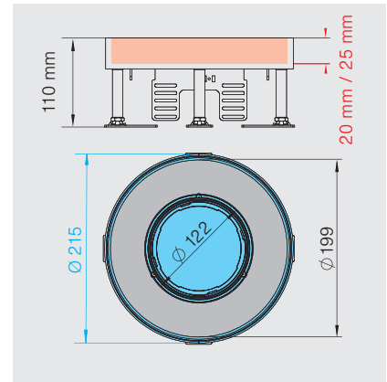
Nenngröße R4, Typ RKFR2 und RKFRN2
