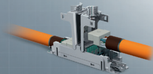
fixlink® Extender Kat. 6 A ISO/IEC CKEF0000 (AWG 24-22) CKEFFLFL (AWG 27-26)
