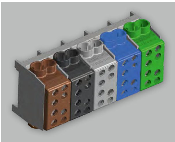
Hauptleitungs-Abweigeklemme, 5-polig main terminal, 5-pole bloc de jonction, 5 pôle
