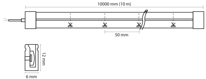
Schéma technique
