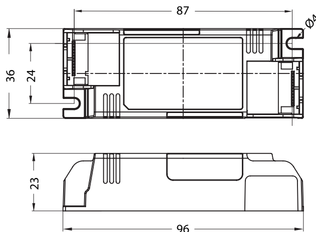
Schéma technique
