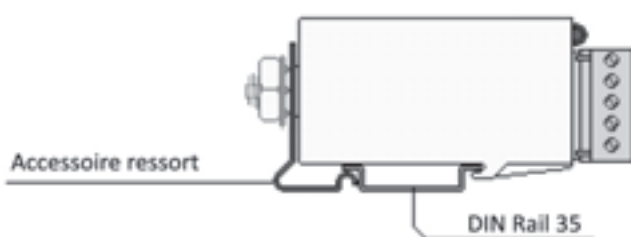
Accessoire pour montage par clipsage
