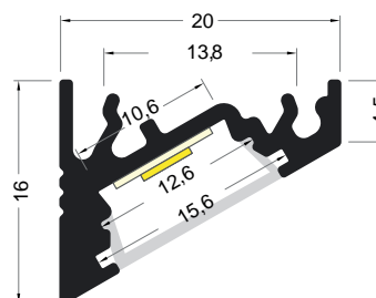
Schéma technique
