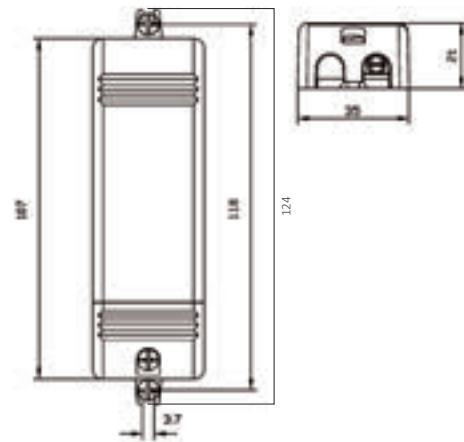
Schéma technique
