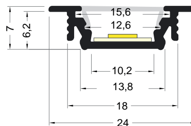
Schéma technique
