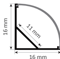
Schéma technique
