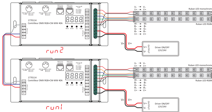
Schémas de câblage
