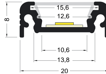
Schéma technique
