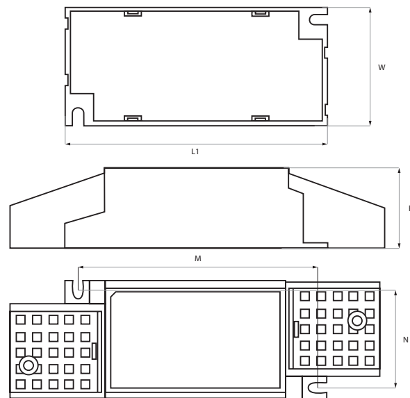
Schéma technique
