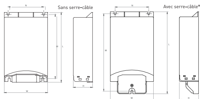
Schéma technique
