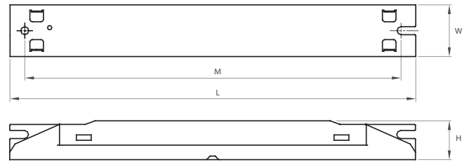
Schéma technique
