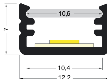
Schéma technique
