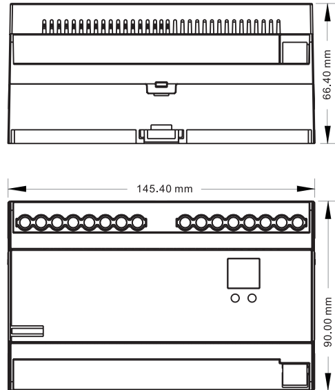
Schéma technique
