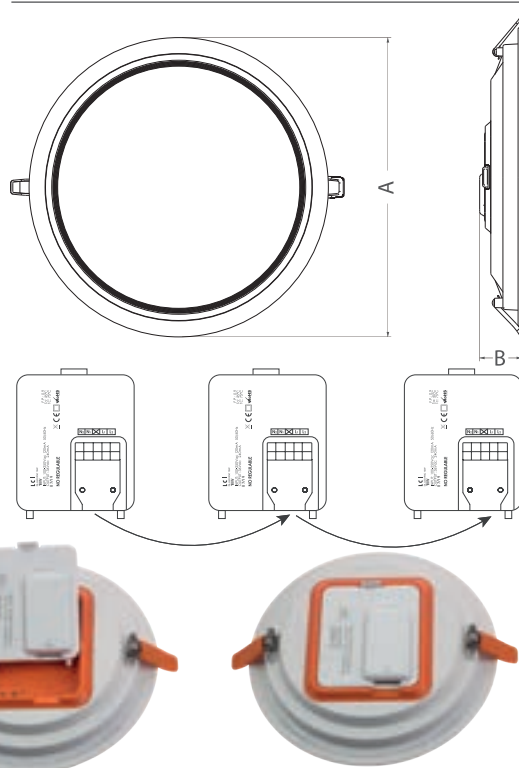
Schéma technique
