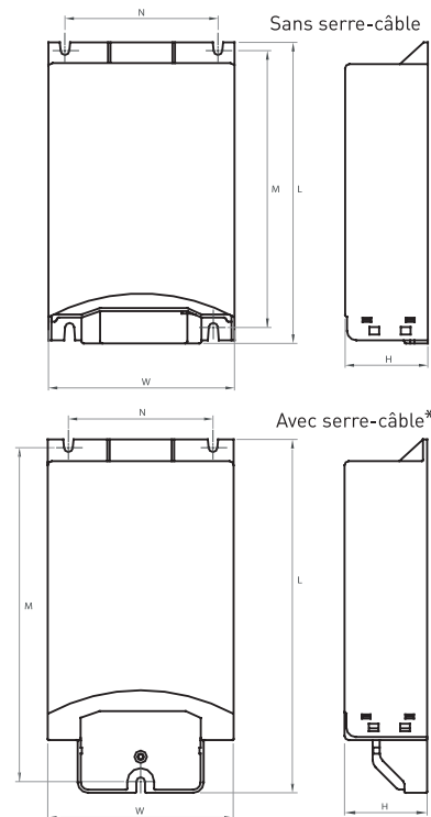
Schéma technique
