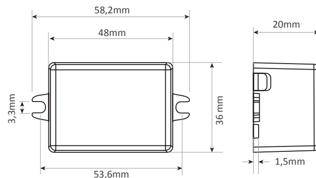
Schéma technique
