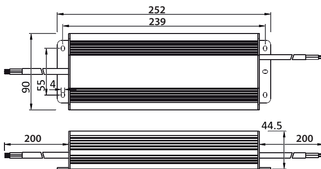
Schéma technique
