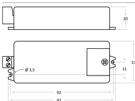
Schéma technique
