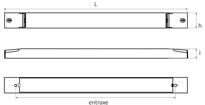
Schéma technique
