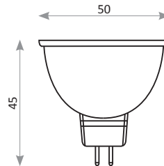
Schéma technique
