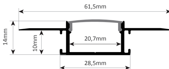
Schéma technique
