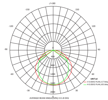
Distribution de l'intensité lumineuse
