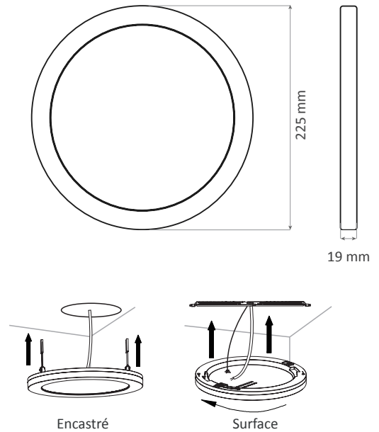
Schéma technique
