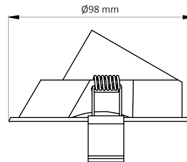
Schéma technique
