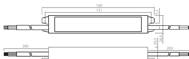
Schéma technique
