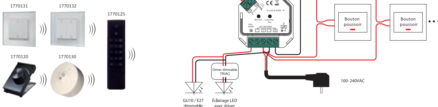
Schéma de câblage
