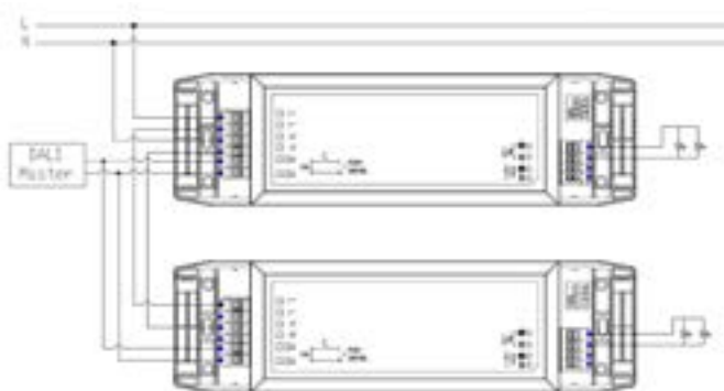
DALI Dim
