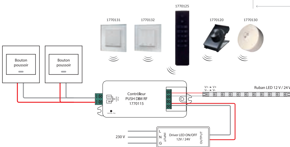
Schéma de câblage
