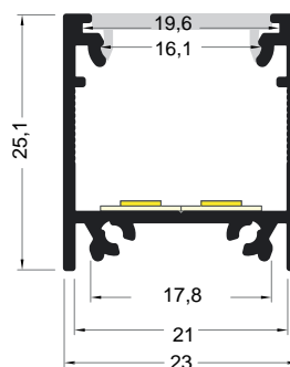
Schéma technique
