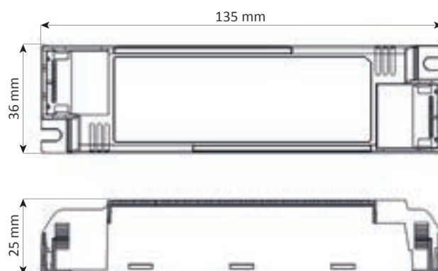
Schéma technique
