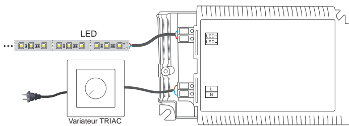
Schéma de câblage
