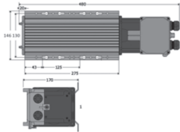
Schéma technique
