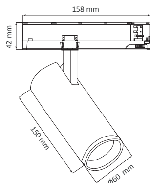
Schéma technique
