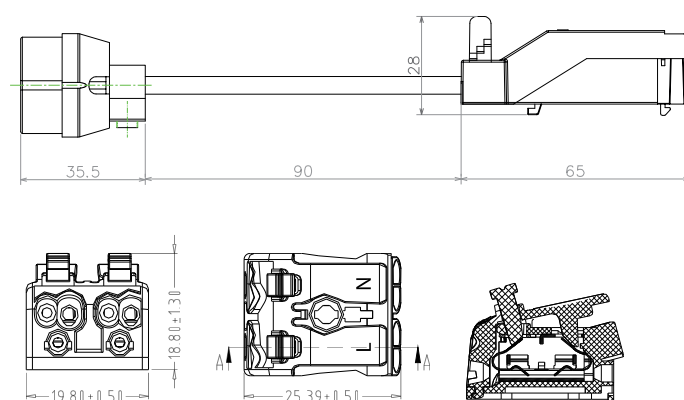
Schéma technique
