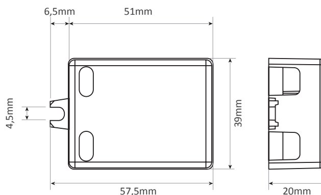
Schéma technique
