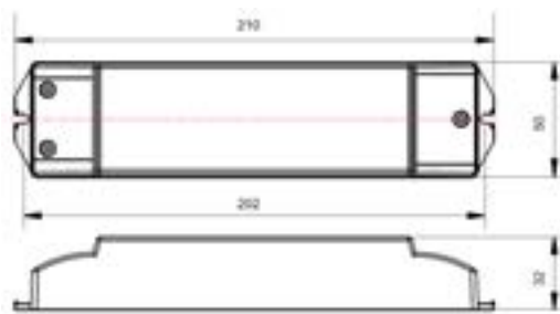
Schéma technique
