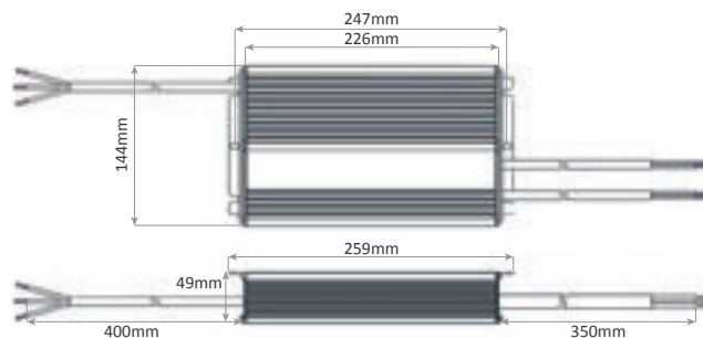
Schéma technique
