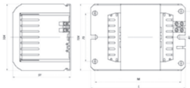
Schéma technique
