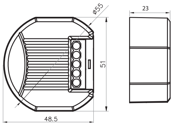
Schéma technique
