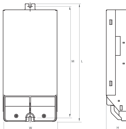
Schéma technique
