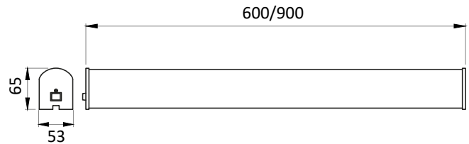
Schéma technique
