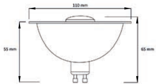
Schéma technique
