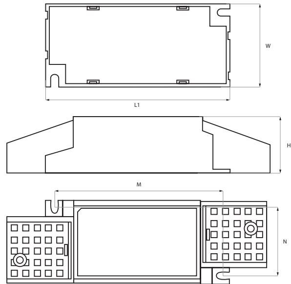
Schéma technique
