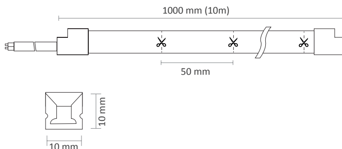
Schéma technique
