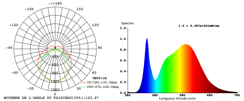
Distribution de l'intensité lumineuse
