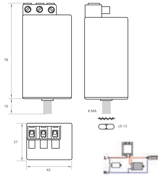
Schéma technique
