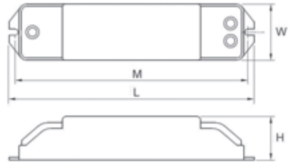
Schéma technique
