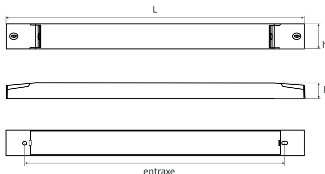
Schéma technique
