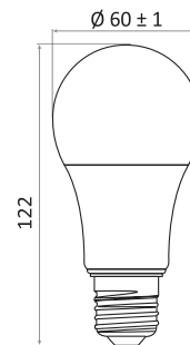
Schéma technique
