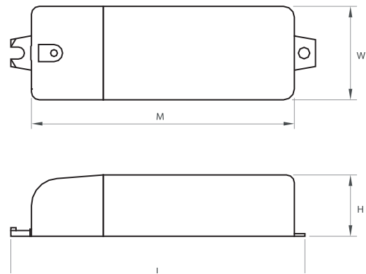
Schéma technique
