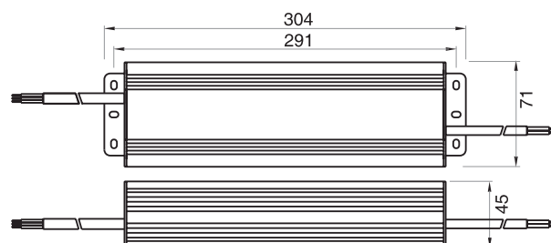
Schéma technique
