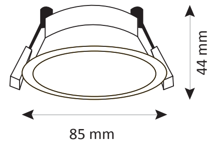
Schéma technique
