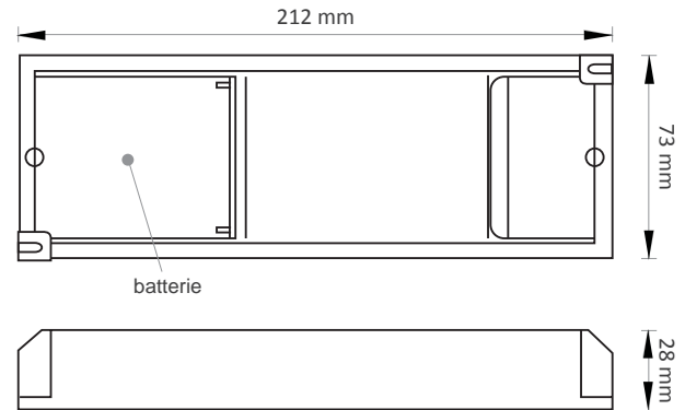
Schéma technique
