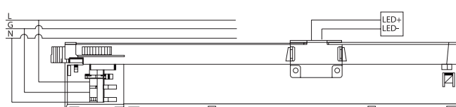
Schéma de câblage
