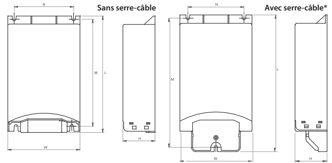
Schéma technique
