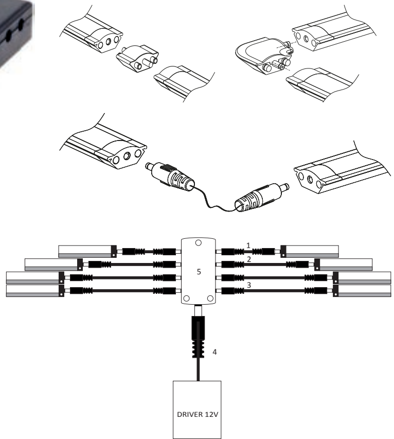
Schéma
