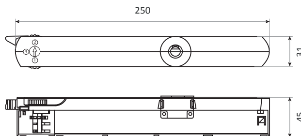
Schéma technique
