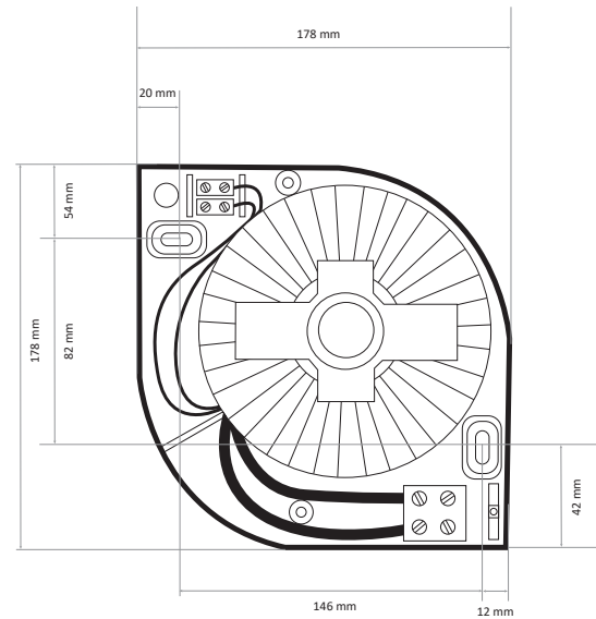
Schéma technique
