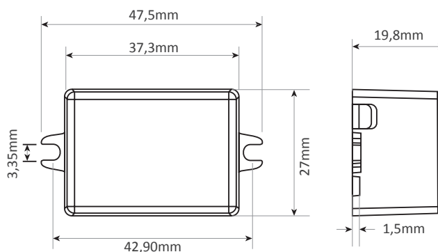
Schéma technique
