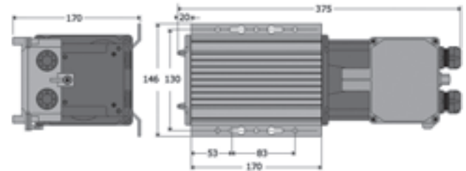
Schéma technique
