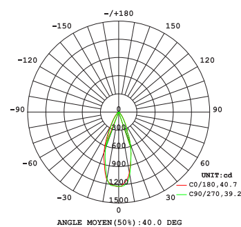
Distribution de l'intensité lumineuse
