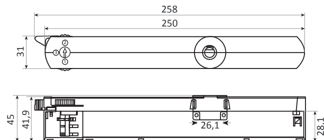
Schéma technique
