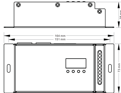
Schéma technique
