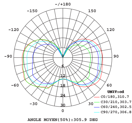
Distribution de l'intensité lumineuse
