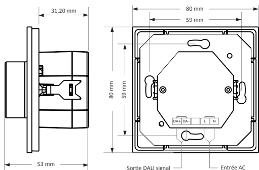
Schéma technique
