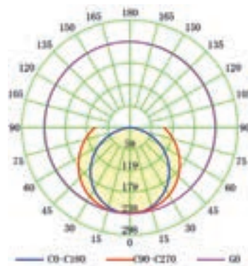
Distribution de l'intensité lumineuse
