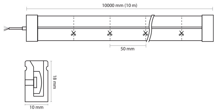
Schéma technique
