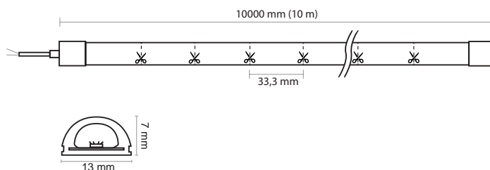
Schéma technique
