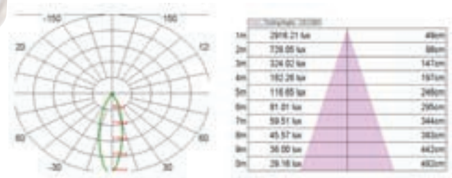
Distribution de l'intensité lumineuse et distance d'illumination
