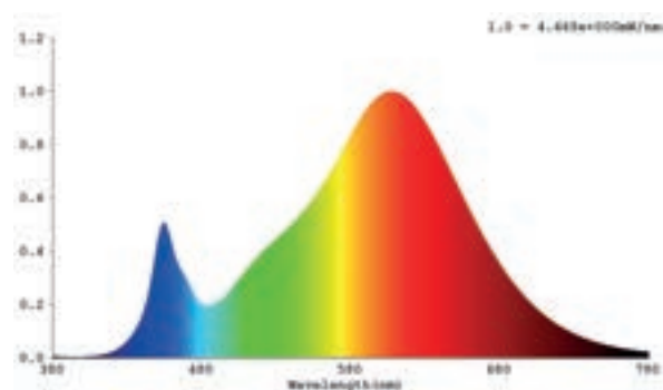
Répartition spectrale
