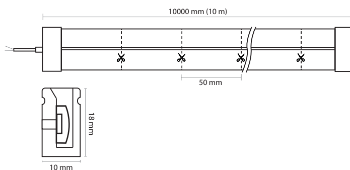
Schéma technique
