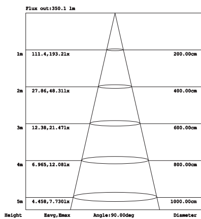
Distance d'illumination
