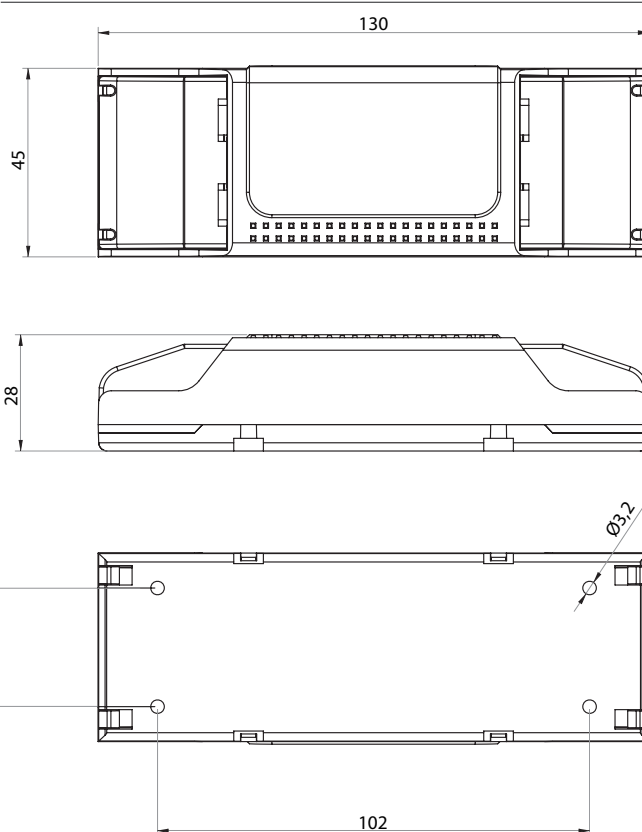
Schéma technique
