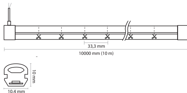
Schéma technique
