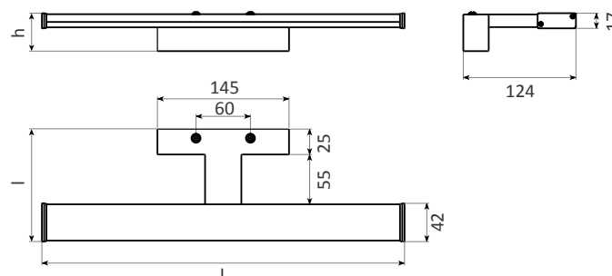
Schéma technique
