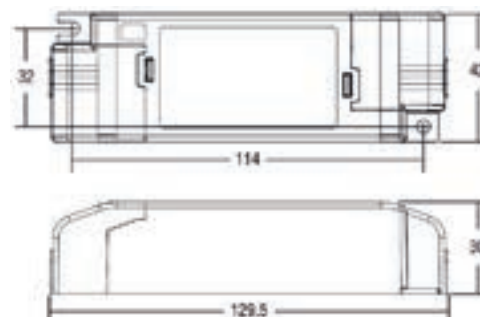
Schéma technique
