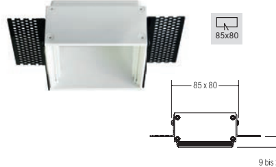
Einputzrahmen quadratisch, für rahmenlosen Einbau
