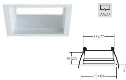
Einbaurahmen, quadratisch
