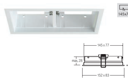
Doppel-Einbaurahmen, rechteckig
